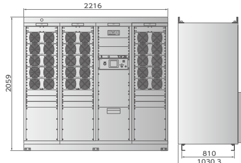
● CRD-2000Q
