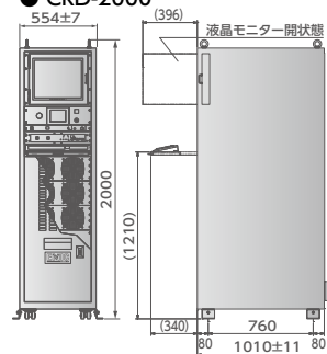
● CRD-2000Q
