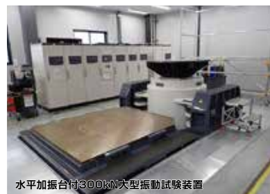
水平加振台付300kN大型振動試験装置
